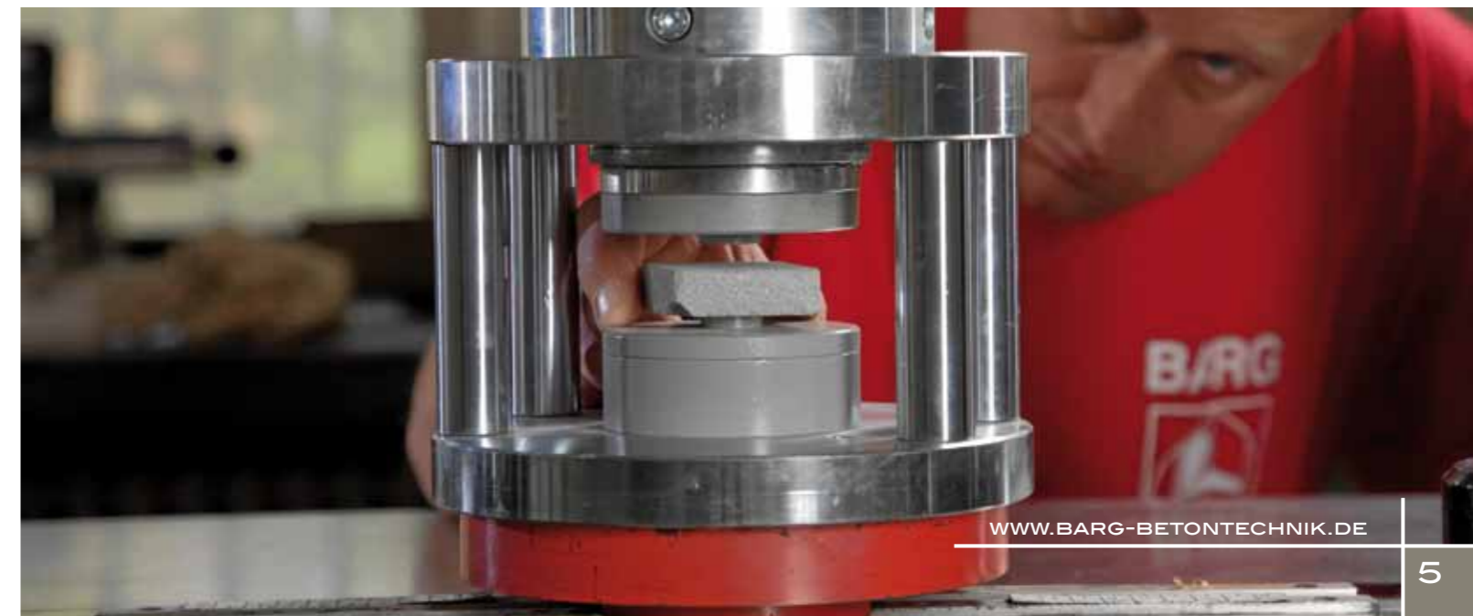
Prüfung der Druckfestigkeit einer Mörtelprobe
